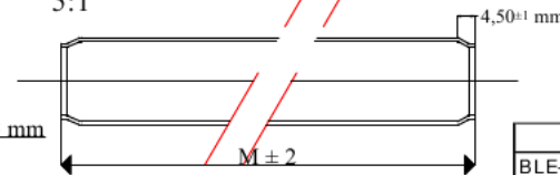
TUBE DETAIL : 5:1
