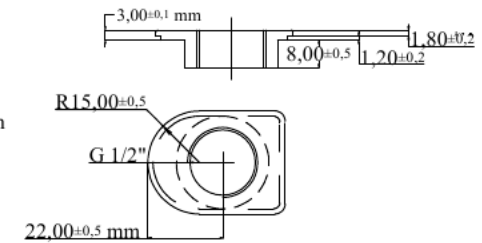
CAP DETAIL : 5:1
